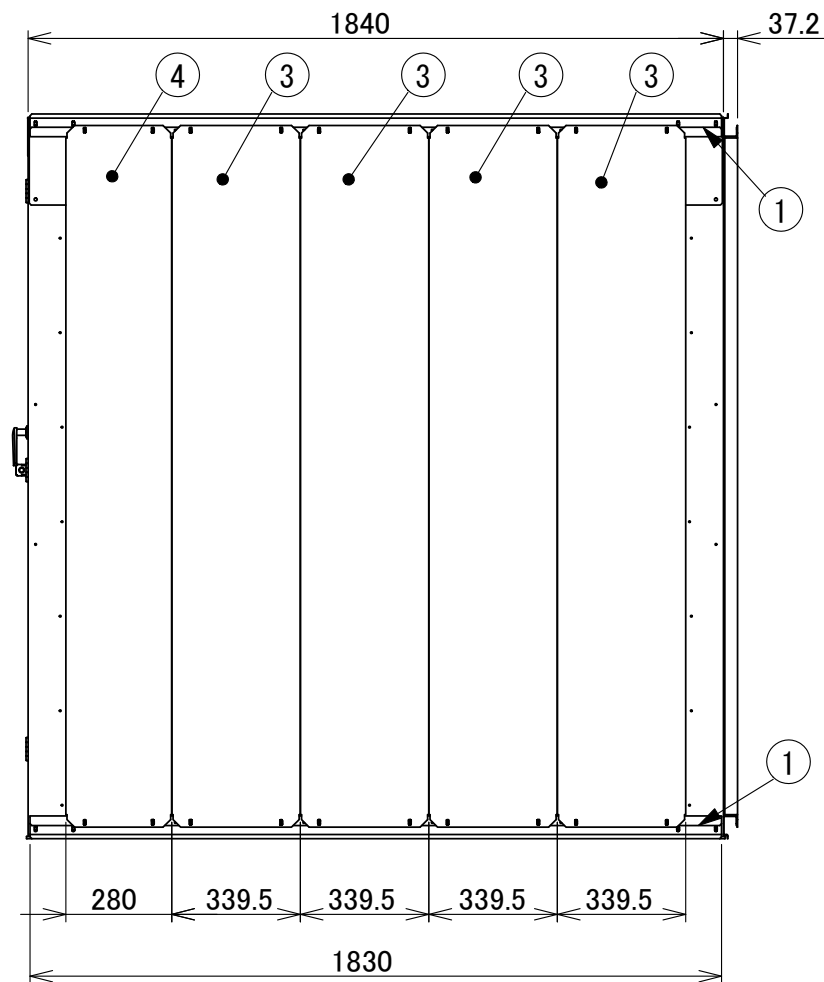
1840用隔壁パネル
