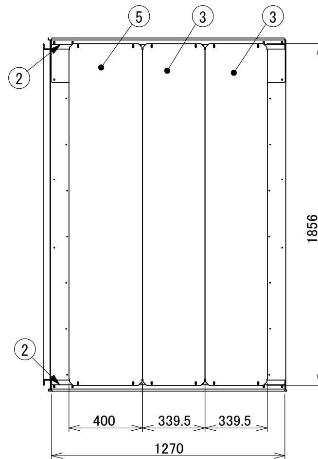
1280用隔壁パネル
